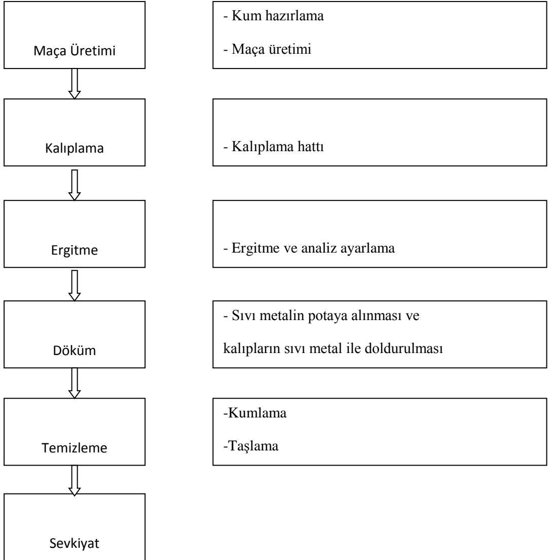
Şekil 2. Döküm Prosesi İş Akış Şeması
